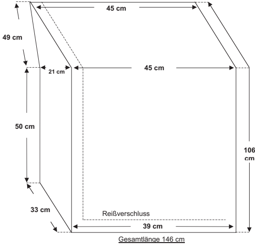
Maßblatt Beinschutzdecke: Universalgröße
