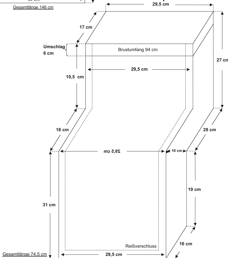
Maßblatt Schlupfsack: Kind 1
